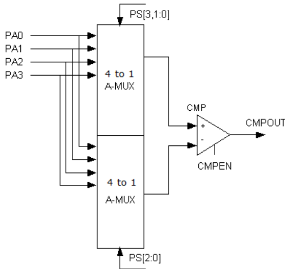
图 33 比较器P2P模式结构框图
