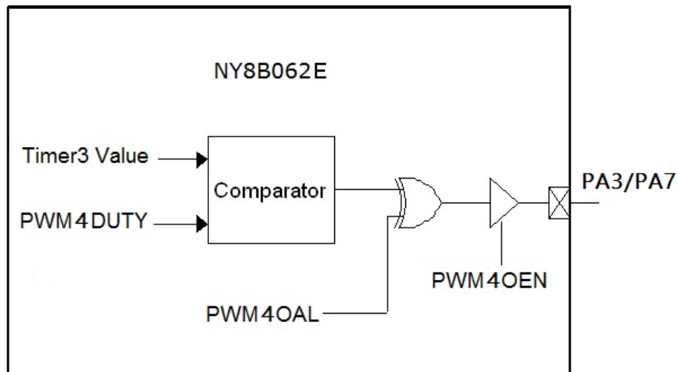
图 28 PWM4 结构框图
