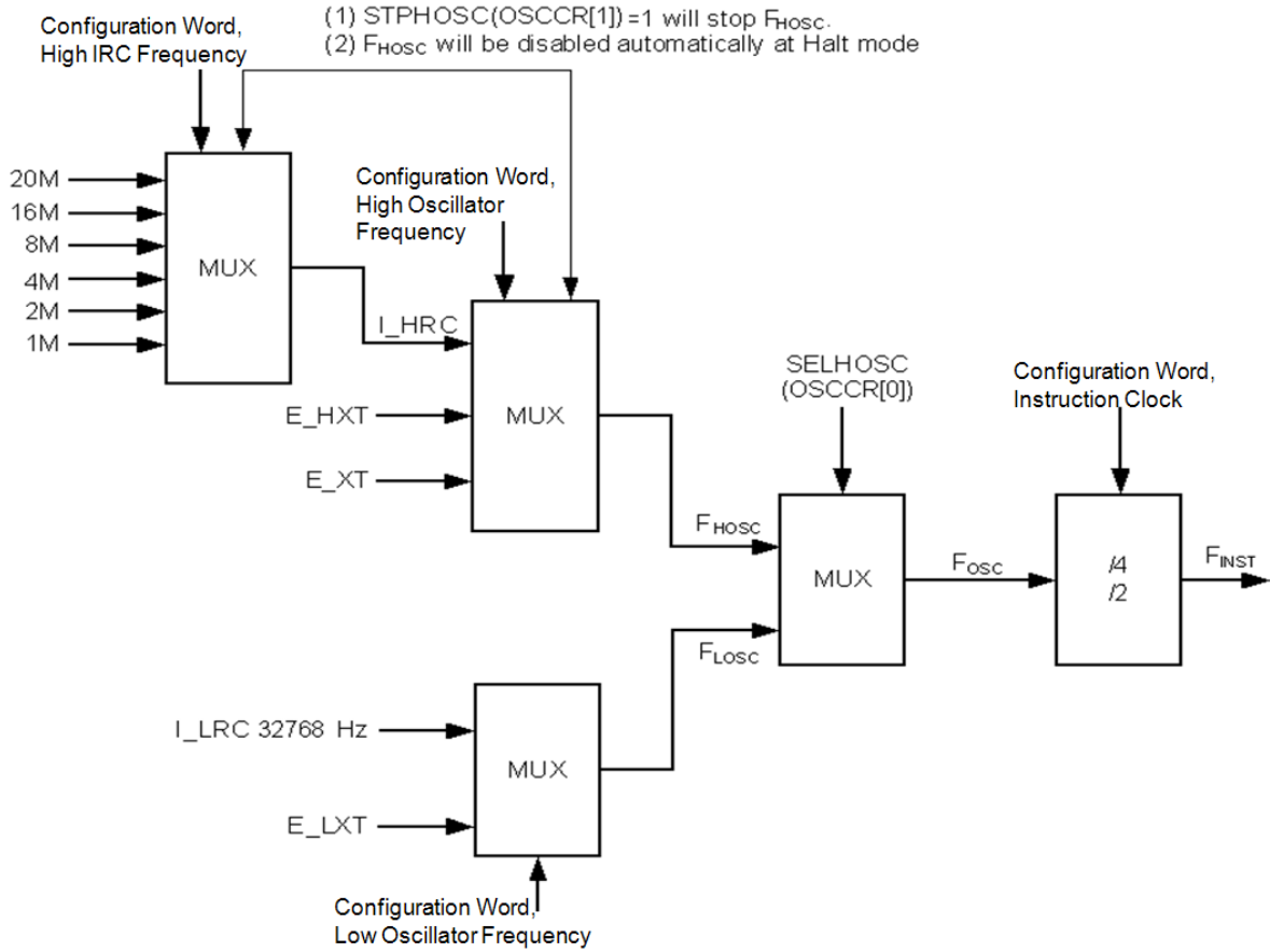
图 35 NY8B062E振荡配置结构图
