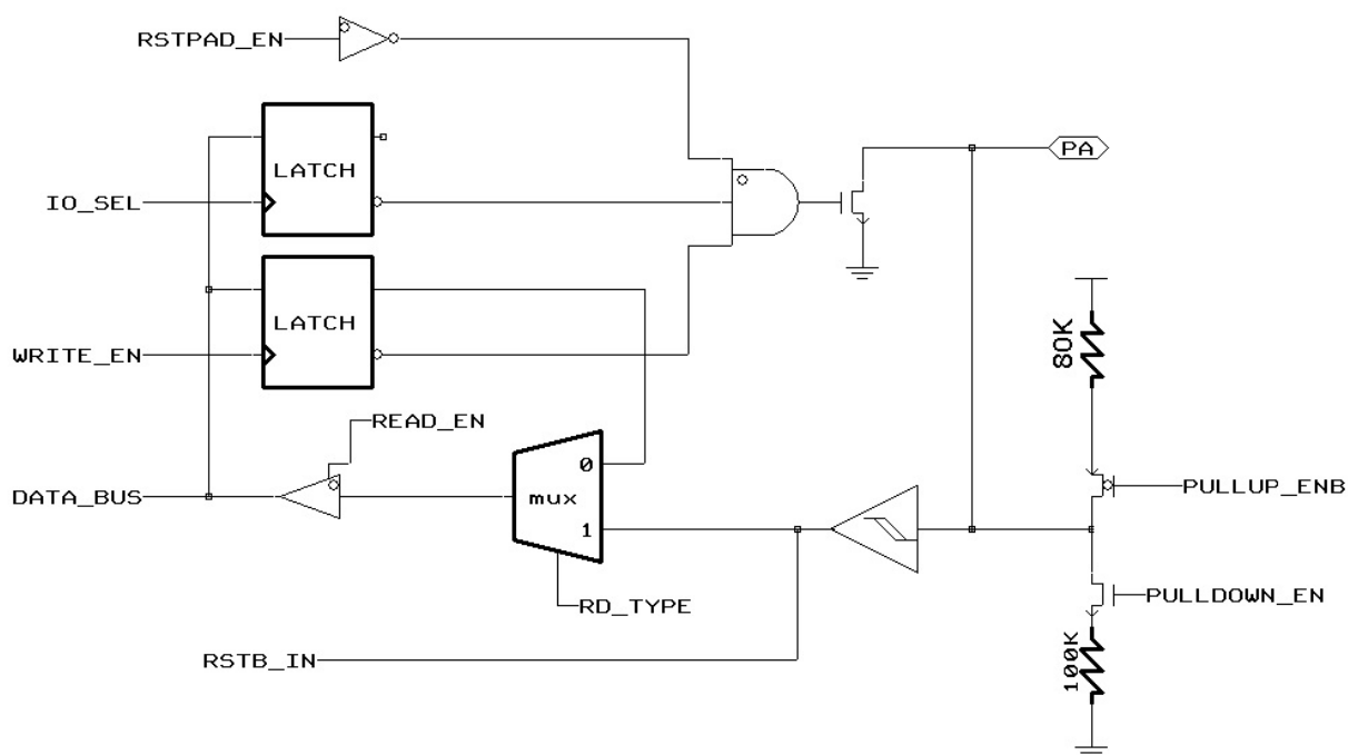
图 8 PA5 引脚结构框图
