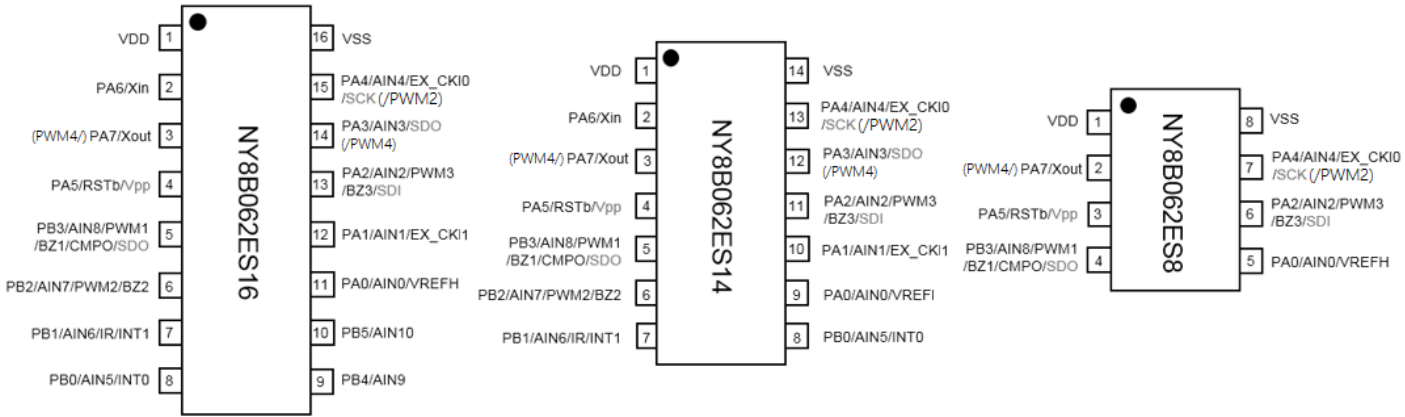
图 1 封装引脚图
