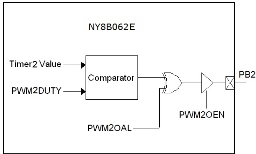
图 22 PWM2 结构框图
