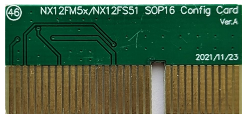
NX12FM5x/NX12FS51 SOP16 转卡 (Config Card)
