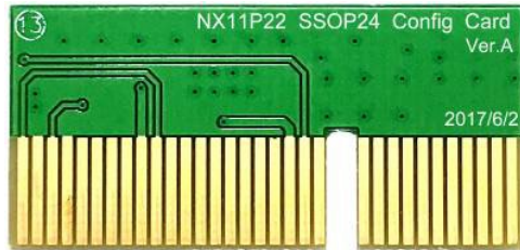
NX11P22 SSOP24 转卡 (Config Card)
