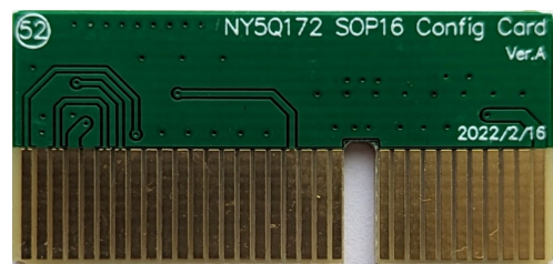
NY5Q172 SOP16 转卡 (Config Card)
