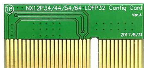
NX12P34/44/54/64 LQFP32 转卡 (Config Card)
