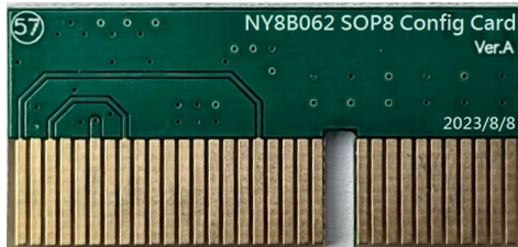
NY8B062 SOP8 转卡 (Config Card)
