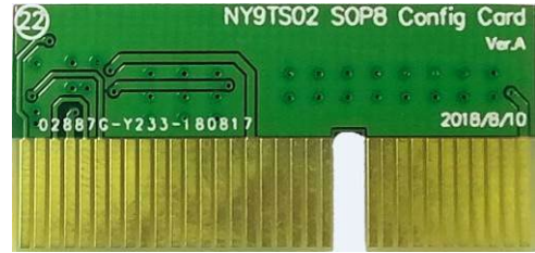
NY9TS02 SOP8 转卡 (Config Card)
