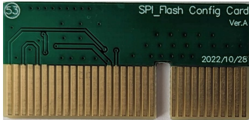
SPI_Flash SOP8 转卡 (Config Card)
