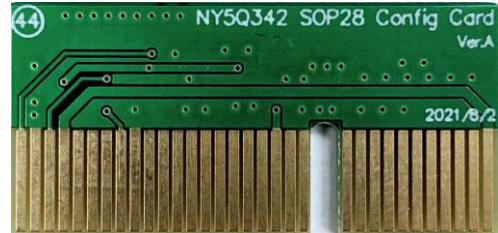
NY5Q342 SOP28 转卡 (Config Card)
