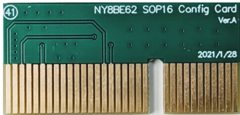
NY8BE62 SOP16 转卡 (Config Card)
