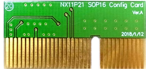
NX11P21 SOP16 转卡 (Config Card)
