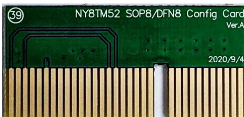
NY8TM52 SOP8/DFN8/COB 转卡 (Config Card)
