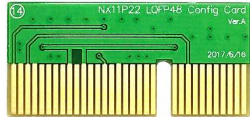
NX11P22 LQFP48 转卡 (Config Card)
