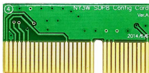
NY3W SOP 转卡 (Config Card)
