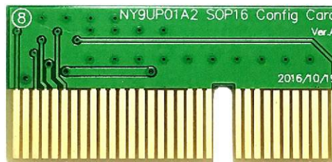
NY9UP01A2 SOP16 转卡 (Config Card)
