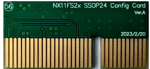
NX11FS2x SSOP24 转卡 (Config Card)
