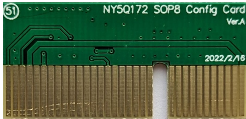
NY5Q172 SOP8 转卡 (Config Card)
