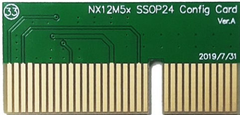
NX12M5x SSOP24 转卡 (Config Card)
