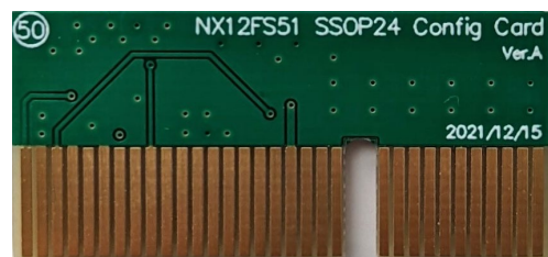
NX12FS51 SSOP24 转卡 (Config Card)
