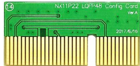
NX11P22 LQFP48 轉卡 (Config Card)
