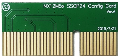
NX12M5x SSOP24 轉卡 (Config Card)
