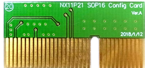
NX11P21 SOP16 轉卡 (Config Card)
