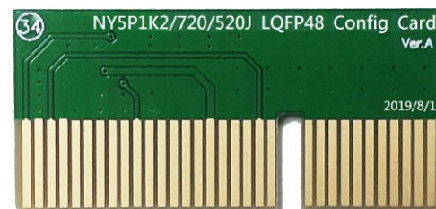
NY5P1K2/720/520J LQFP48 轉卡 (Config Card)
