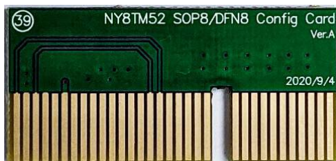
NY8TM52 SOP8/DFN8/COB 轉卡 (Config Card)
