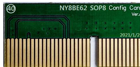
NY8BE62 SOP8 轉卡 (Config Card)
