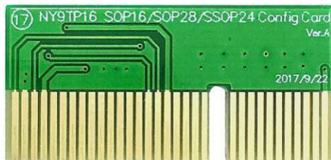
NY9TP16 SOP16/SOP28/SSOP24 轉卡 (Config Card)
