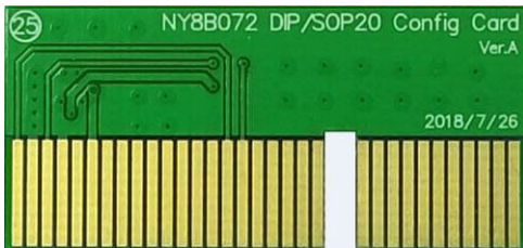
NY8B072 DIP/SOP20 轉卡 (Config Card)
