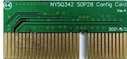
NY5Q342 SOP28 轉卡 (Config Card)
