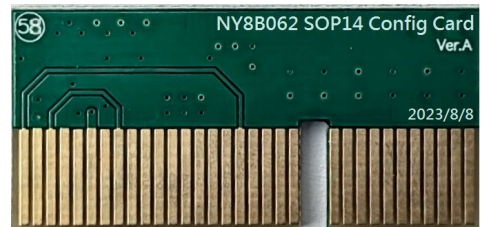
NY8B062 SOP14 轉卡 (Config Card)
