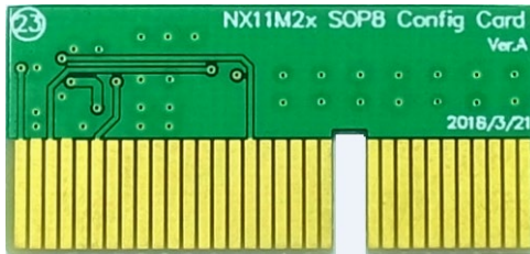
NX11M2x SOP8 轉卡 (Config Card)
