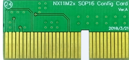
NX11M2x SOP16 轉卡 (Config Card)
