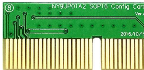
NY9UP01A2 SOP16 轉卡 (Config Card)
