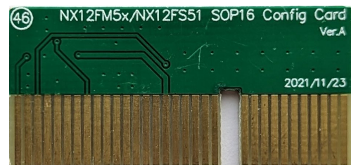
NX12FM5x/NX12FS51 SOP16 轉卡 (Config Card)
