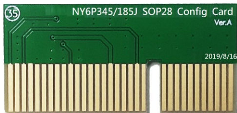
NY6P345/185J SOP28 轉卡 (Config Card)
