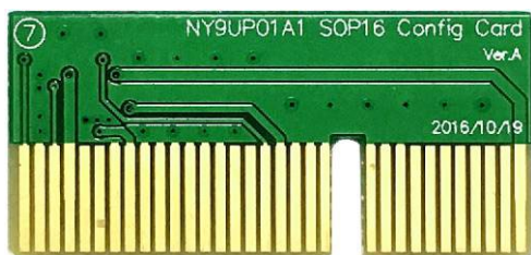
NY9UP01A1 SOP16 轉卡 (Config Card)
