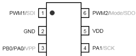
SOT23-6
