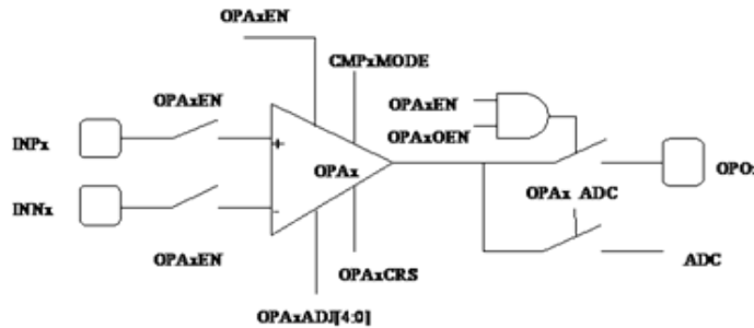
Figure 53 OPAx BLOCK(OPAxOEN SW->OPAxEN & OPAxOEN)
