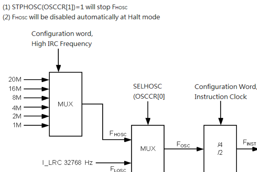
图 18 NY8A051H振荡配置结构图
