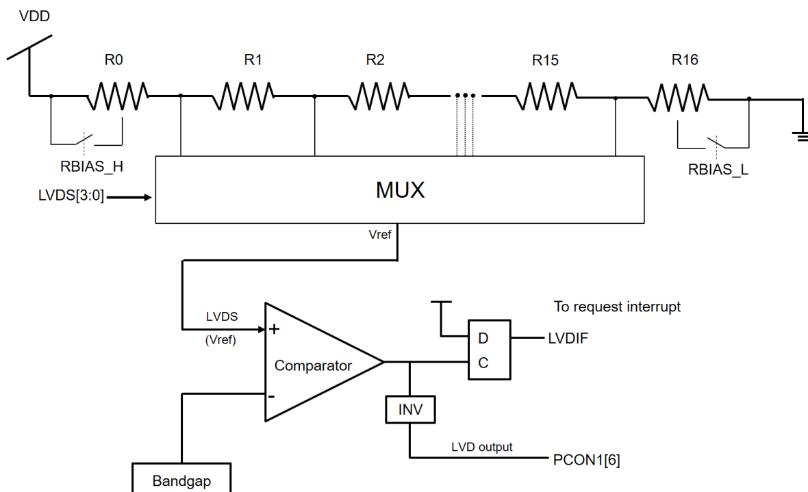
圖 17 Vref硬件连接及LVD结构框图
