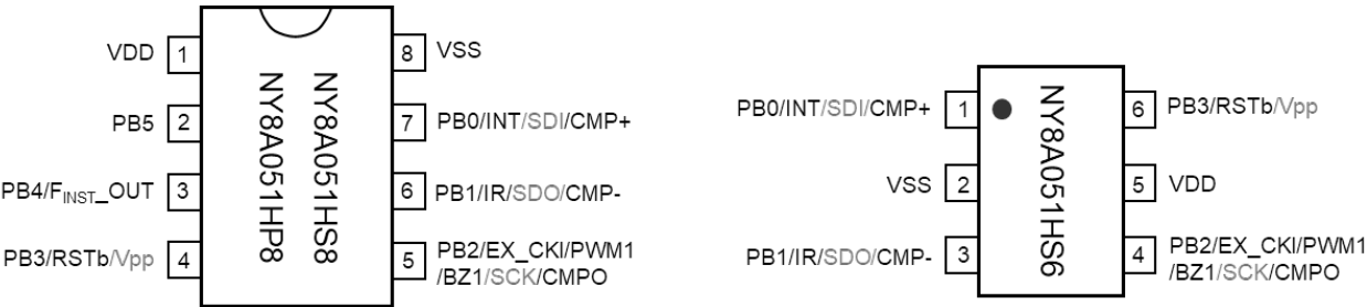
图 1 封装引脚图
