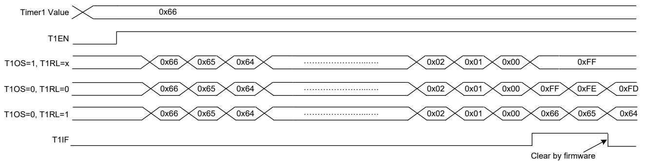
图 12 定时器T1 时序图
